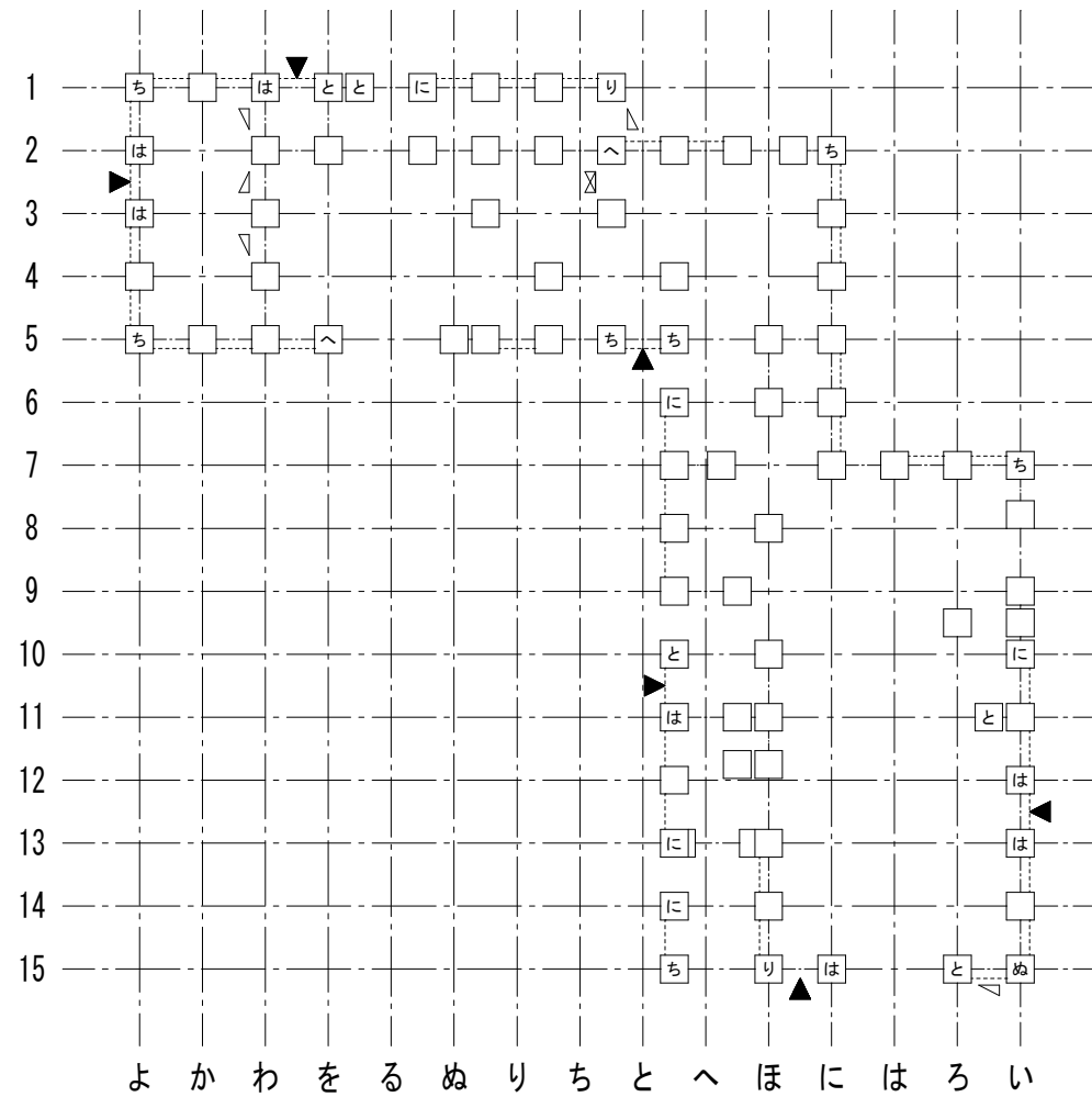
1 階柱壁伏図
