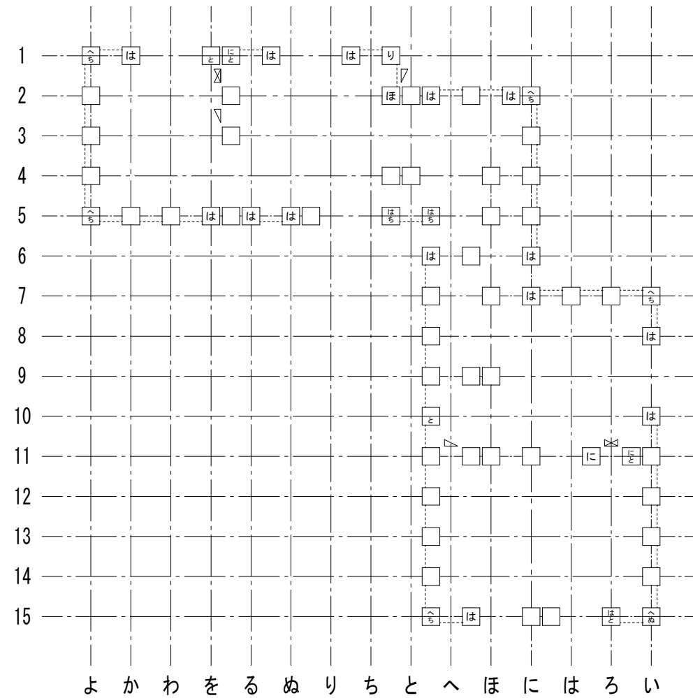
2 階柱壁伏図
